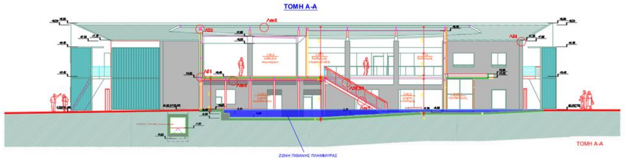
Σχέδιο 2 : Τομή Α-Α Ισογείου
