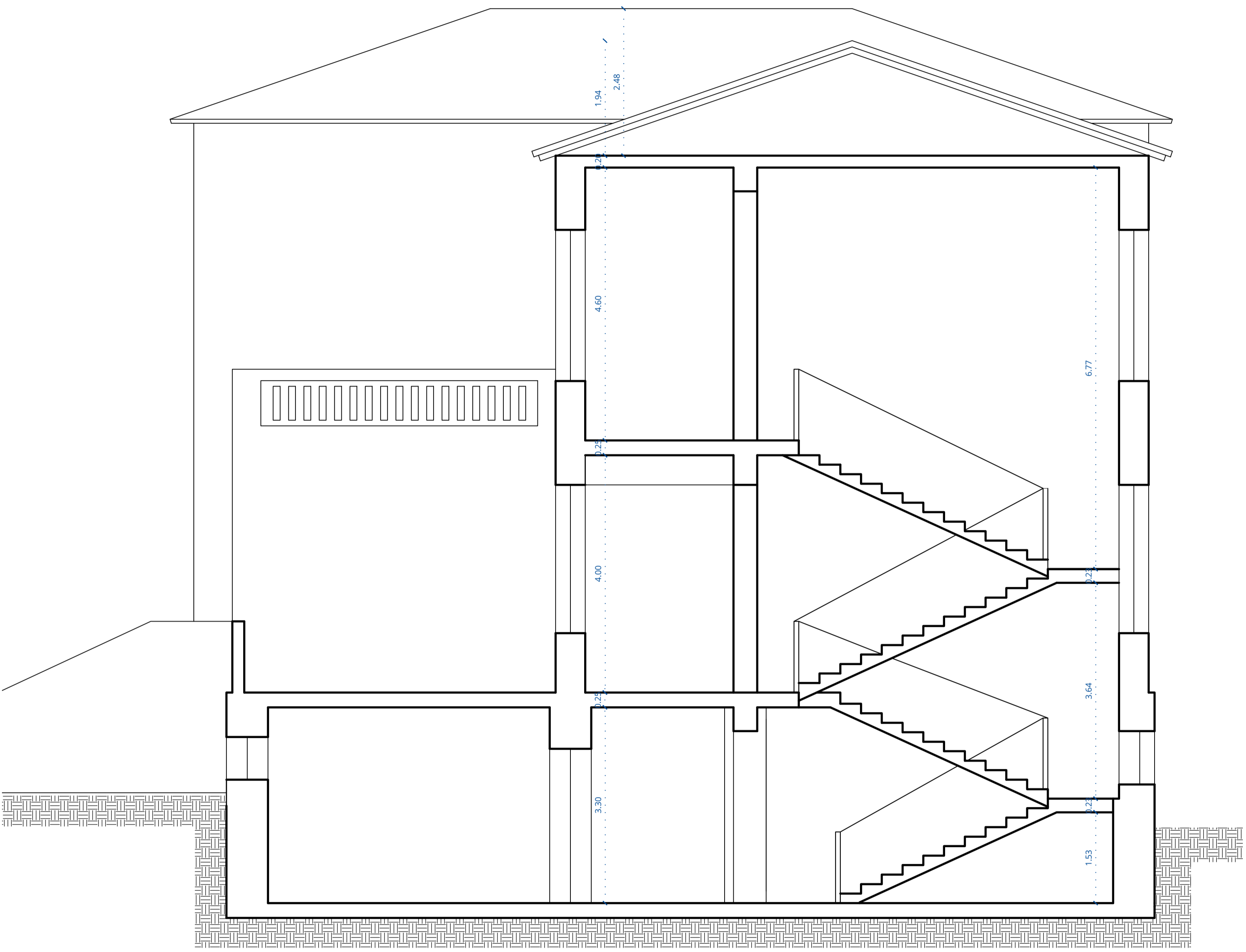
ΣΧΗΜΑΤΙΚΗ ΤΟΜΗ Α-Α ΚΛΙΜΑΚΑ 1:50
