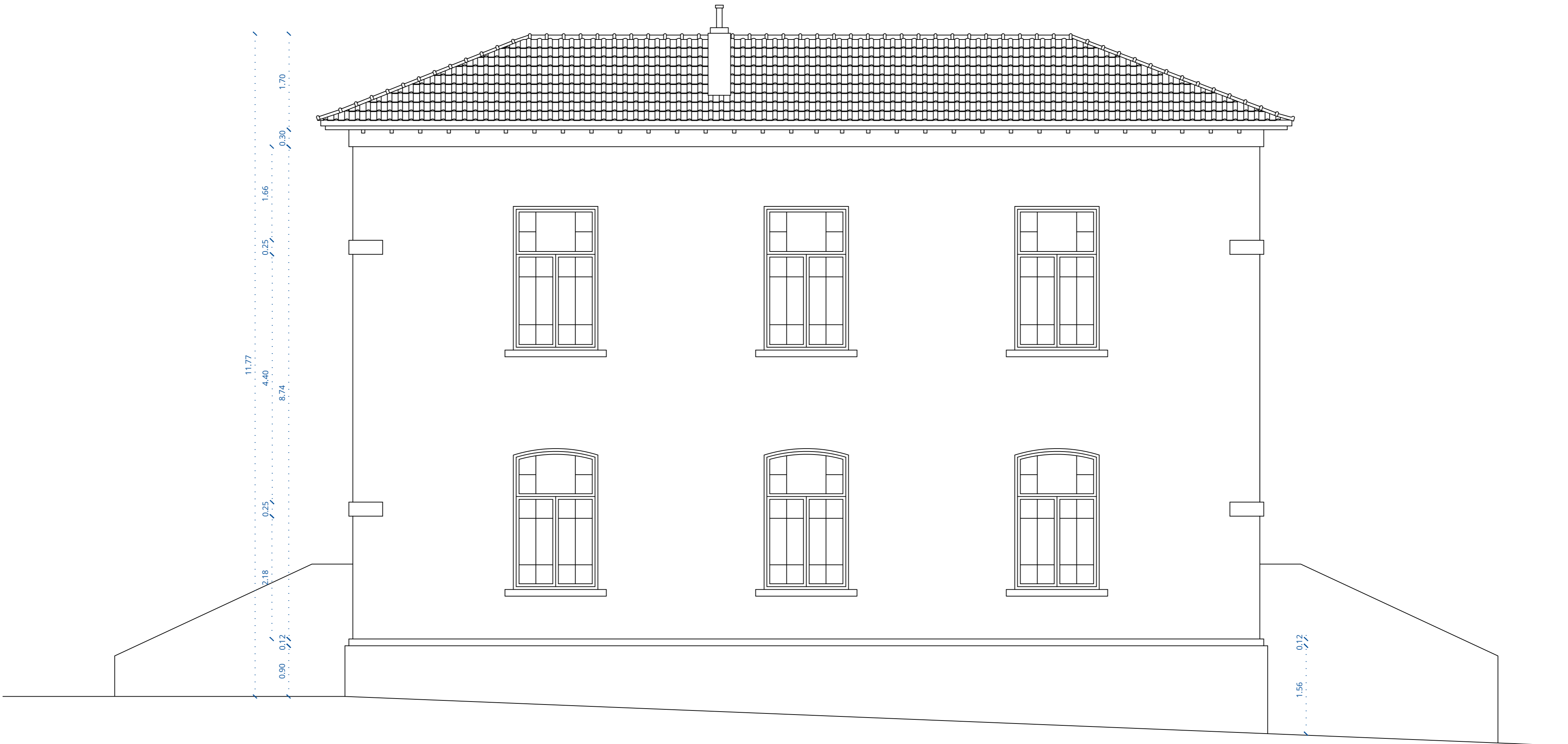
ΔΥΤΙΚΗ ΟΨΗ ΚΛΙΜΑΚΑ 1:50
